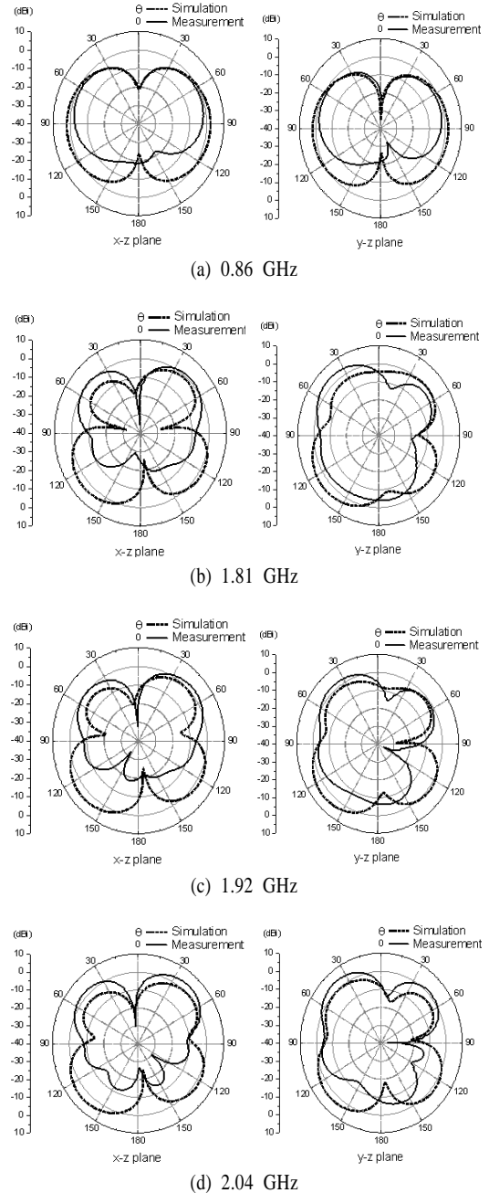
그림 8. 제안한 안테나의 x-z, y-z 평면에서의 복사 패턴 Fig. 8. Measured radiation patterns of the proposed antenna in the x-z and y-z plane.
