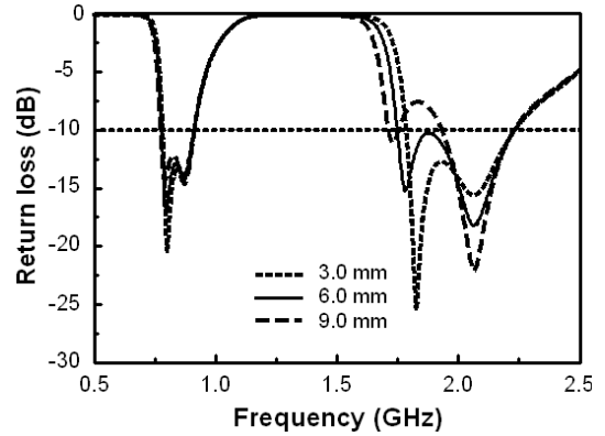
그림 5. 슬릿 길이 변화에 따른 반사 손실 Fig. 5. Variation of return loss with respect to the length of slit.
