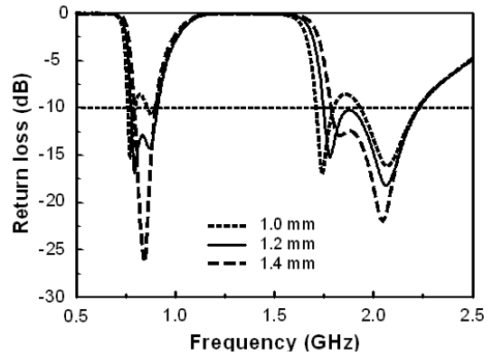
그림 3. 상부 사각 스파이럴 라인의 간격 변화에 따른 반사 손실
